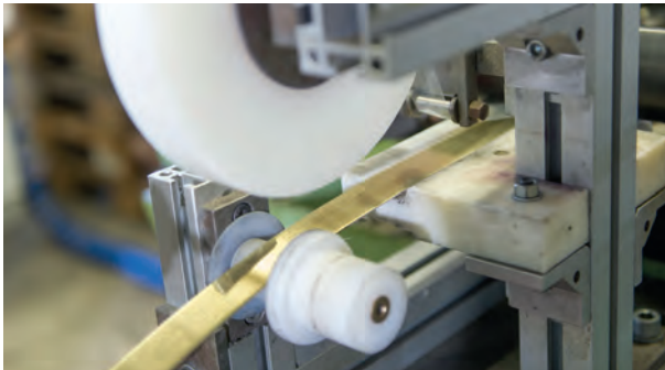
Profilbearbeitungsanlage Section processing plant
